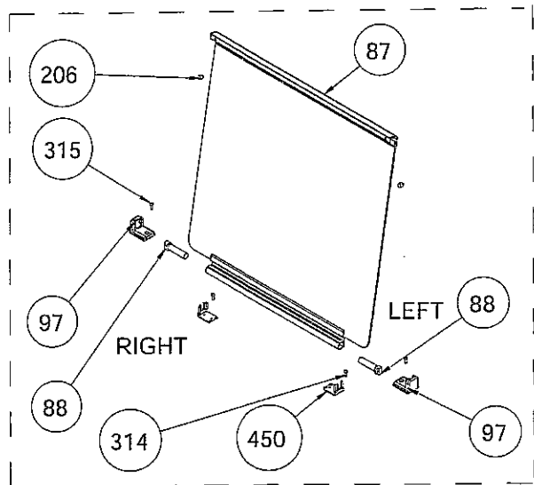
GLASS LID OPTIONAL
